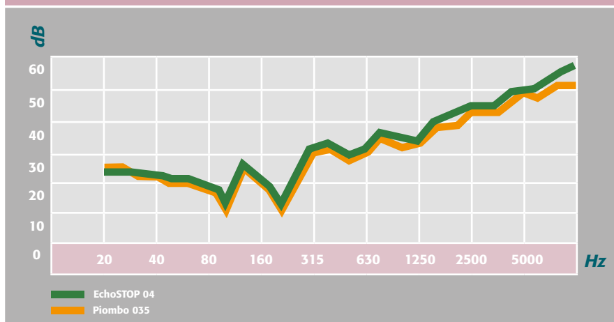
Confronto potere fonoisolante EchoSTOP 04 (4 kg/m 2 ) - Piombo 035 (4 kg/m 2 )
